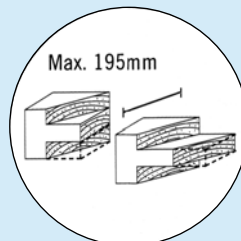
Mitred Tenon
